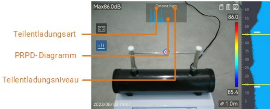
Teilentladungsanzeige
