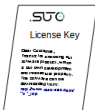
LMS-Lizenzschlüssel (x1)
