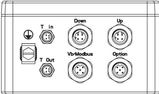
Anordnung der Anschlüsse
