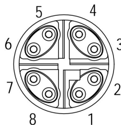
Ethernet-Anschlusspins, männlich (Blick auf den Sensorstecker)
