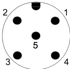
5-polig-Stecker, männlich (Blick auf den Sensorstecker )
